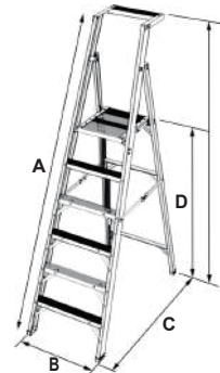
ESCALERA ABIERTA
