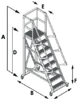
DIMENSIONES
